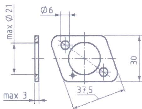
Монтажный план.
