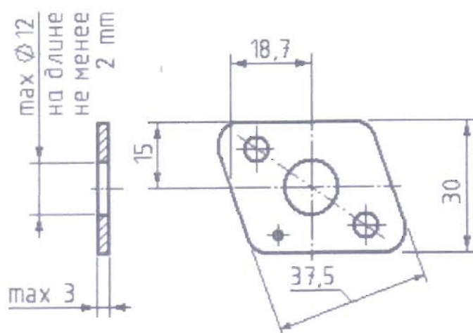
2. Дроссельная шайба.
