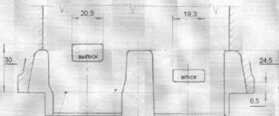
РАЗВЕРТКА ЦИЛИНДРА
